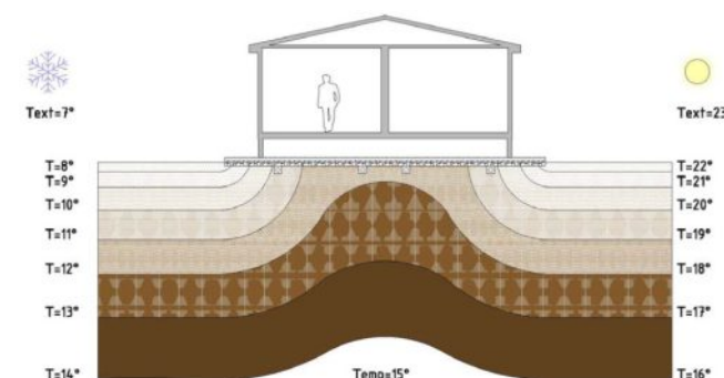
esquema de la gradiente constante bajo la vivienda
